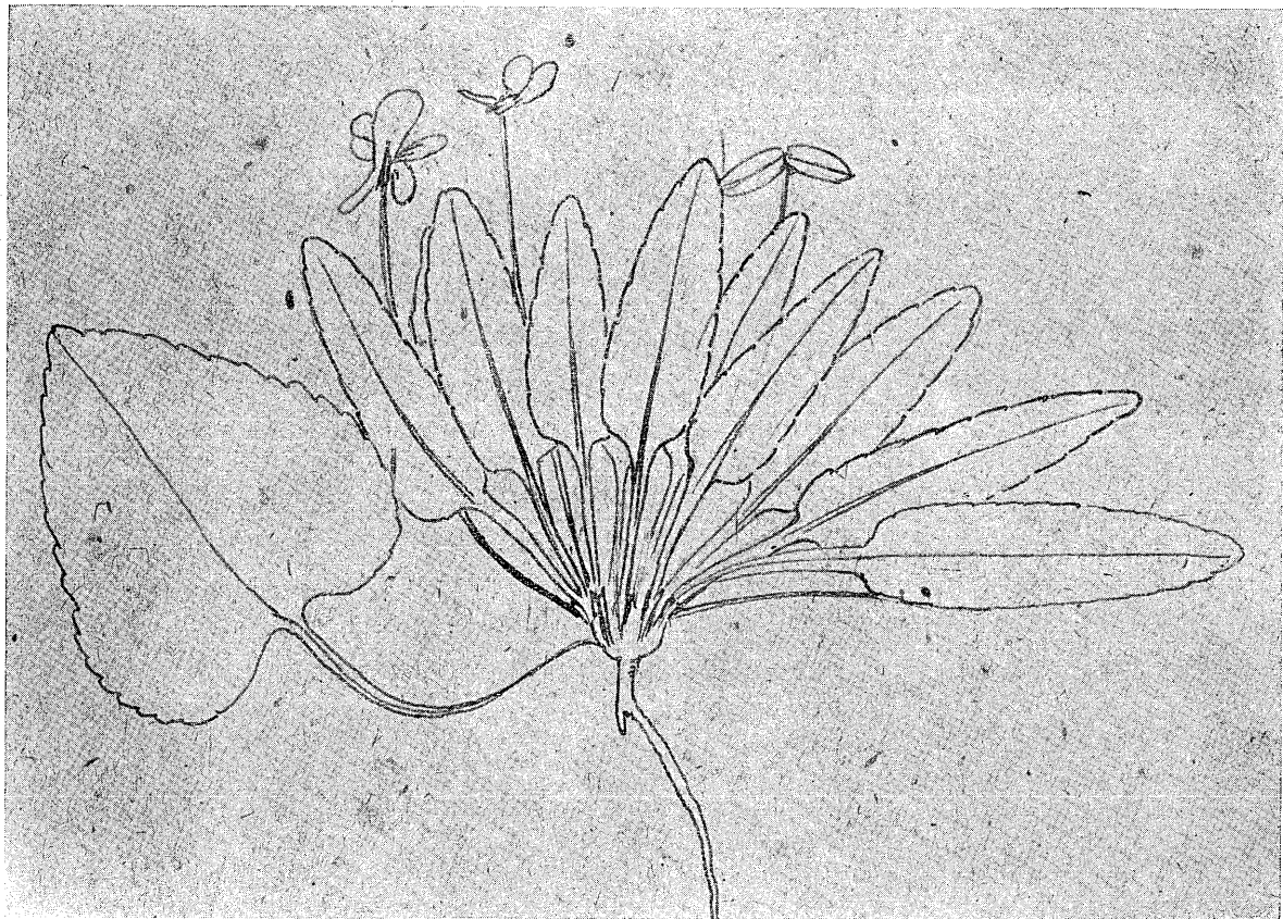
圖解。British MuseumノBANKS herbarium 中ニアル Viola Patrini B. chinensis ノtype specimen ノ寫生圖。 實物大ナレドモ根ノ端ヲ約 6 cm ダケ除ク。
