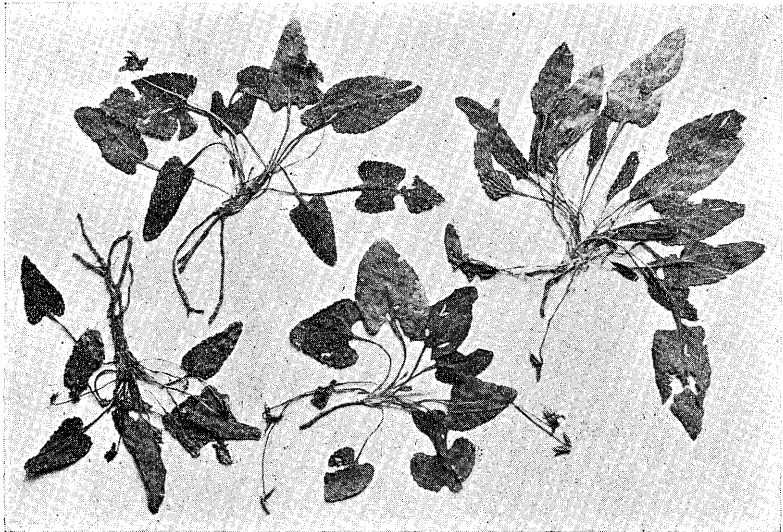
第1圖 V. yedoensis MAKINO, ca. 1/3. (coll. H. MIGO, Shanghai, Dec. 6, 1940).
