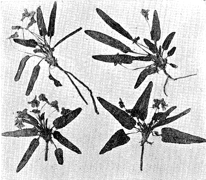
第2圖 V. yedoensis MAKINO, ca. \frac{1}{2} . (coll. H. MIGO, Shanghai, Mar. 20, 1941).
